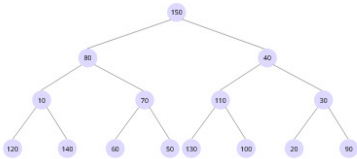
Árbol desordenado
